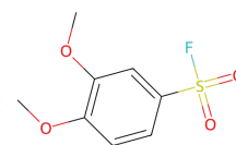
3,4-Dimethoxybenzenesulfonyl fluoride
